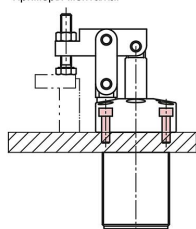
Сверху с четырьмя винтами с цилиндрической головкой через фланец.
