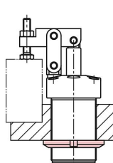
Корпус ввинчивается в резьбовое отверстие и фиксируется шлицевой гайкой.
