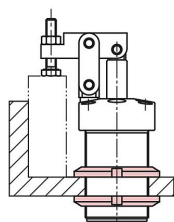
Со шлицевой гайкой сверху и шлицевой гайкой снизу.
