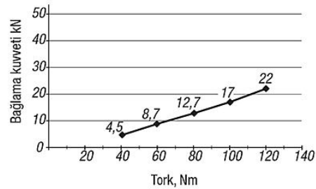
3 akslı bağlama elemanı bağlama kuvveti
